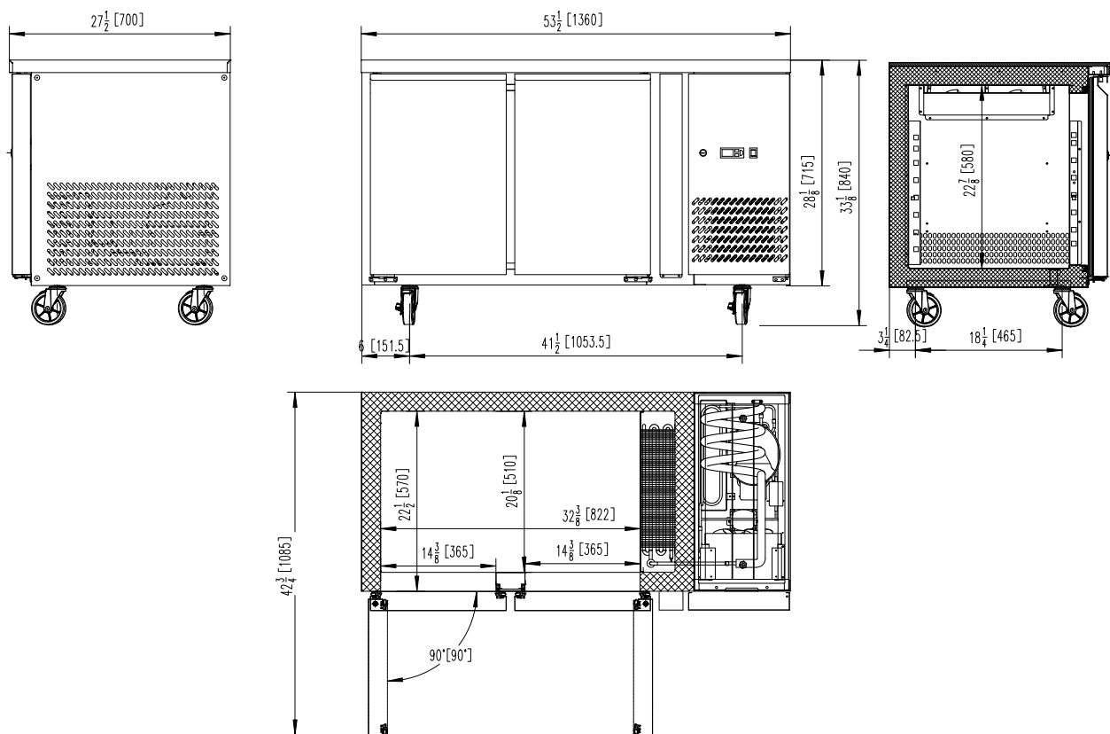
EPF3462GR, 3422GR
